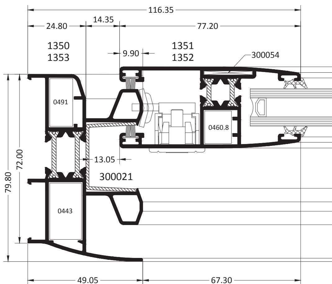
SECCIÓN S3
