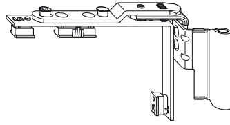
Falso Compás Derecha E13 Ref. 0300-J2D
