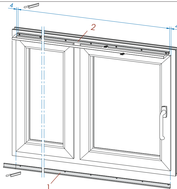
Dibujo 1: Guía (arriba) / Rail (abajo)
