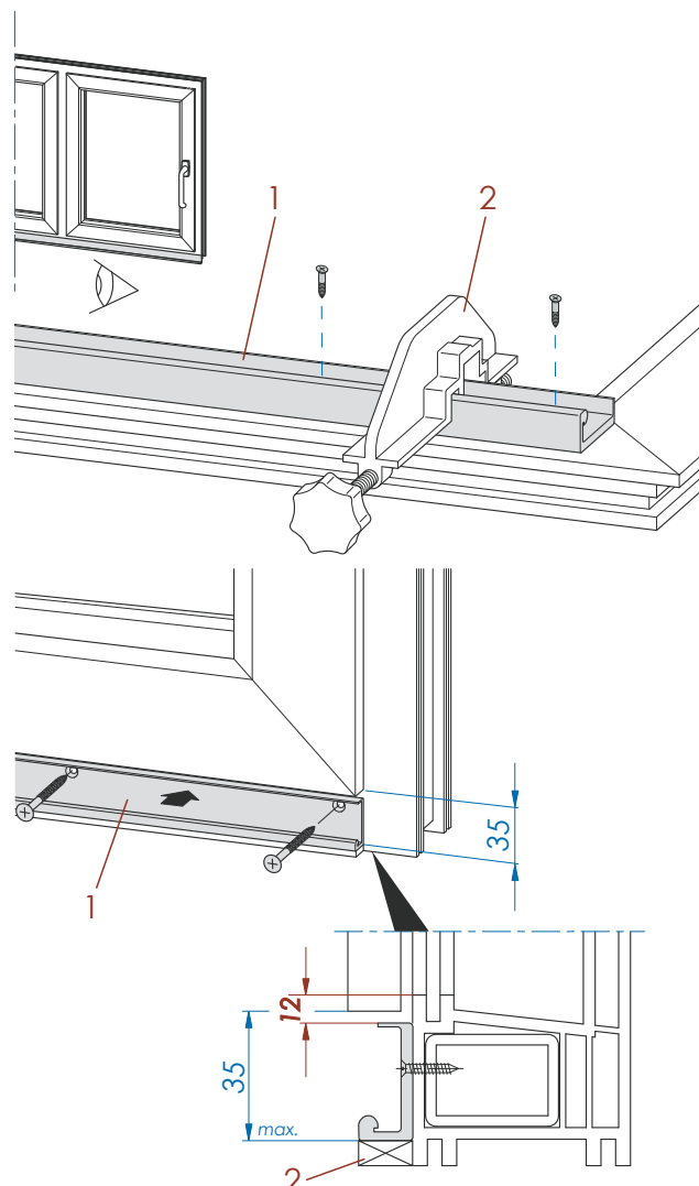
Dibujo 3: Guía inferior. Situación
