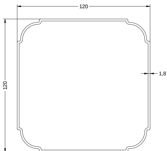
Ref.2668 TUBO DE 120x120 DE PERGOLA
