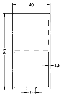
Ref.2471 GUÍA PERGOLA DE 80 MM.
