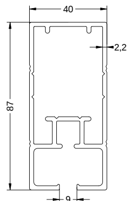
Ref.2460 * GUÍA PERGOLA MOTORIZADA
