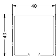
Ref.2472 GUÍA PERGOLA DE 40mm
