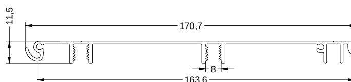
Ref.2493 VISERA PARA TOLDO 170 MM.
